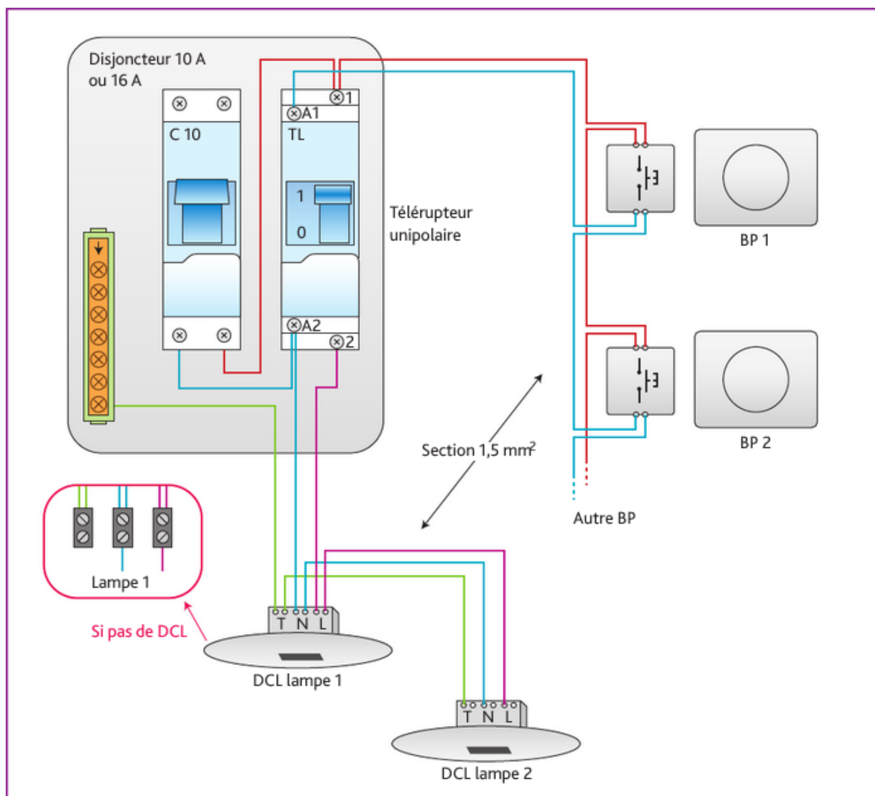
20 Schéma de câblage d'un va-et-vient par télérupteur.
